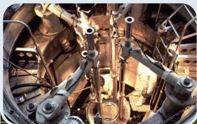
Réacteur expérimental EOLE
